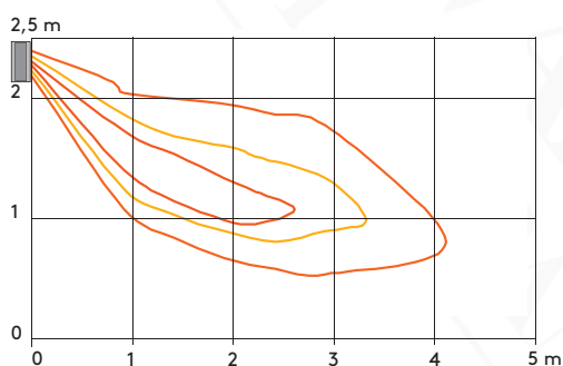
Luftverteilung MIT Komfort-Luftgitter (Wärmeluft wird zum Boden geleitet)
