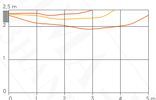
Luftverteilung OHNE Komfort-Luftgitter (Wärmeluft bleibt unter der Decke)
