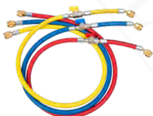
CCL-36-CA-½"-20UNF
